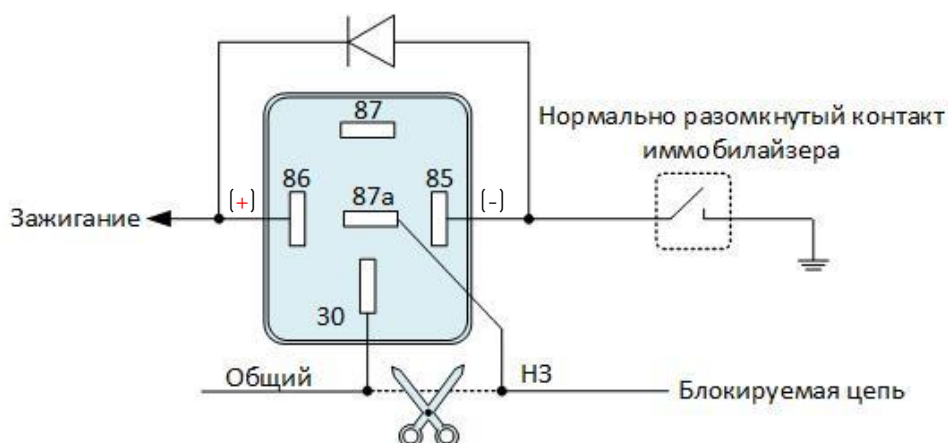
Рисунок Б.4 – Подключение внешнего реле НЗ блокировки
