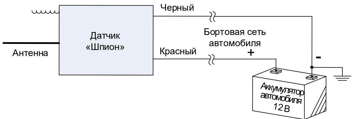
Рисунок Г.2 - Схема подключения Шпион
