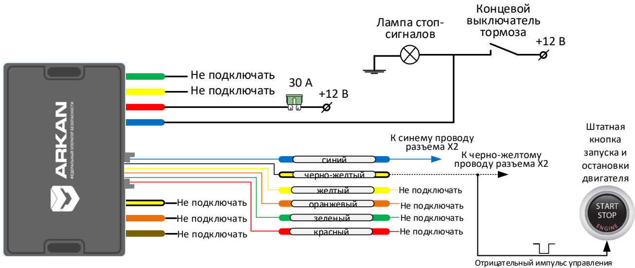
Рисунок Г.1 – Схема подключения Силового модуля автозапуска на автомобилях с кнопкой «Старт-Стоп»
