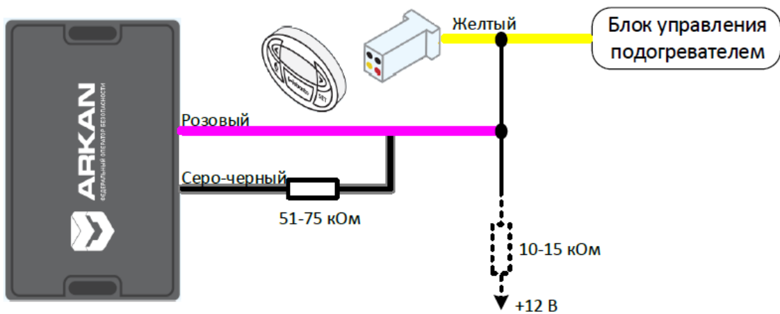
Рисунок В.2 - Схема подключения предпусковых подогревателей Webasto
