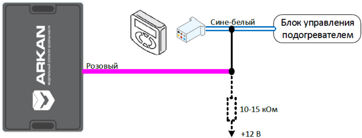
Рисунок В.1 - Схема подключения предпусковых подогревателей Eberspacher
