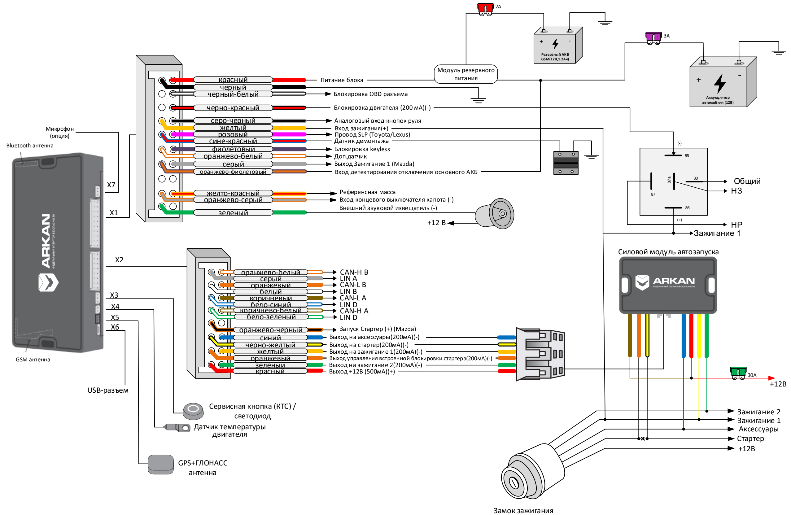
Рисунок А.1 – Схема подключения Комплекса со встроенным CAN-модулем (Тип блокировки программируется через ARKAN Мастер)
