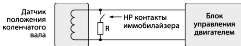
Рисунок Б.3 – Подключение внешнего реле НР блокировки
